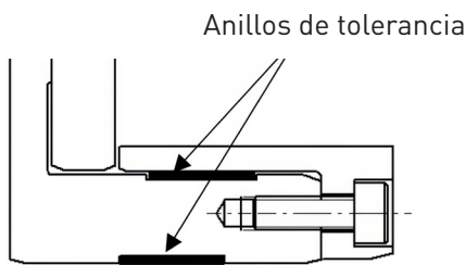
FIGURA 1. CAMISA DE EJE INSTALADA CON FRANJA DE TOLERANCIA
