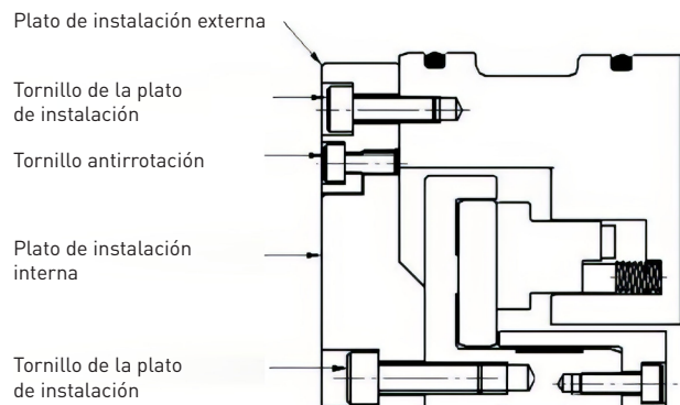
FIGURA 2. SELLO DE SEPARACIÓN CON PLACAS DE INSTALACIÓN COLOCADAS
